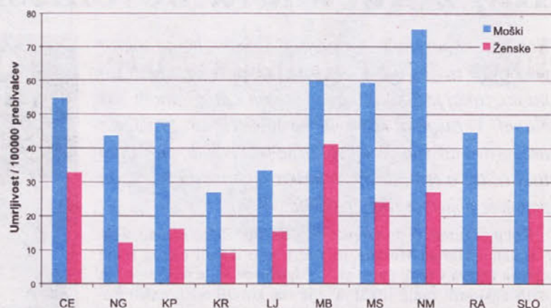
Umrljivost zaradi ciroze jeter po regijah v letih 1991-1996
