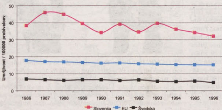
Umrljivost zaradi ciroze jeter, Slovenija, EU in Švedska, 1986-1996
