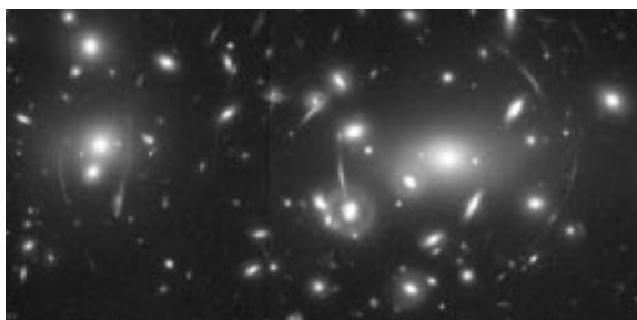
Gravitacijska leča pred skupino galaksij
