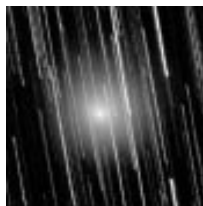
Komet Tempel-Tuttle januarja letos
