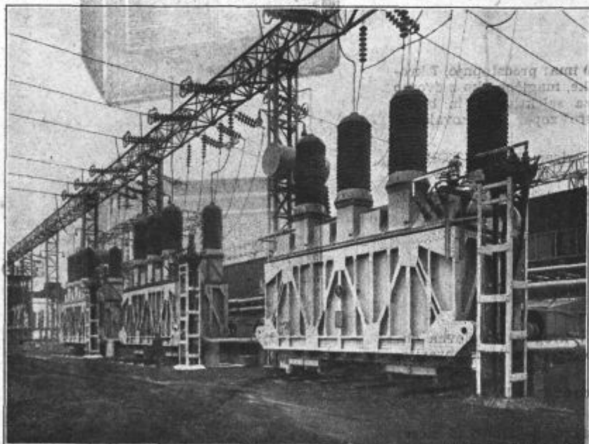
Trije velikanski transformatorji rensko-vestfalske elektrarne pri Kölnu. Vsak tehta 185.000 kg in je 9 m visok.
