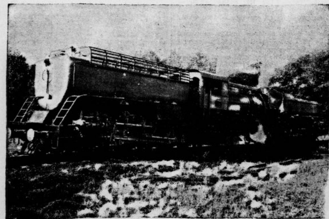
V Roubaixu na Francoskem so izdelali lokomotivo, ki bo vozila v ozemlju Nigra v Afriki. Lokomotiva meri v dolžino 23 m, tehta 150 ton, njena kolesa pa so napravljena za progo, ki ima samo 1 m širine
