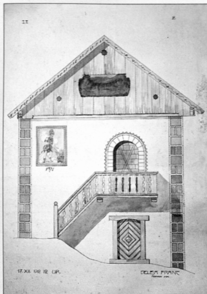
Takole je Franc Deleja, znani tesarski mojster v Mozirju, leta 1912 za svoj mojstrski izpit narisal kaščo.
