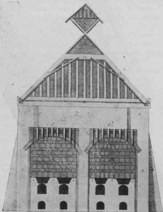
Navpični prerez skozi isto peč
