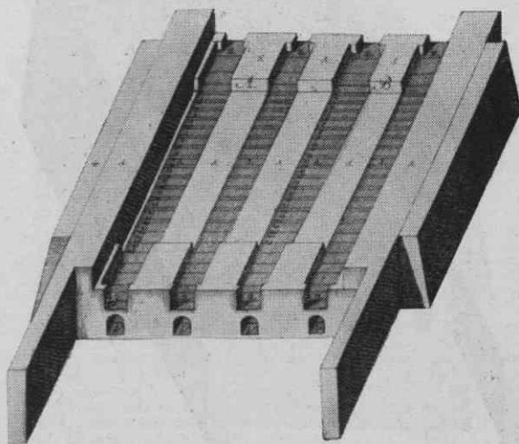
Vodoravni prerez skozi isto peč I.
