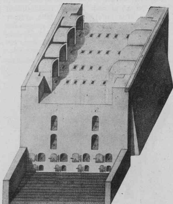
Opekarniška peč na premog — celotni pogled (po brošuri iz l. 1799 med spisi Komisije za požarno brambo; Mestni arhiv v Ljubljani)
