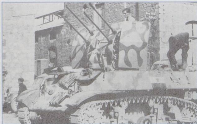
Nemški protiletalski Flak, montiran na tank namesto poškodovane kupole v mehanični delavnici v Šibeniku decembra 1944.
