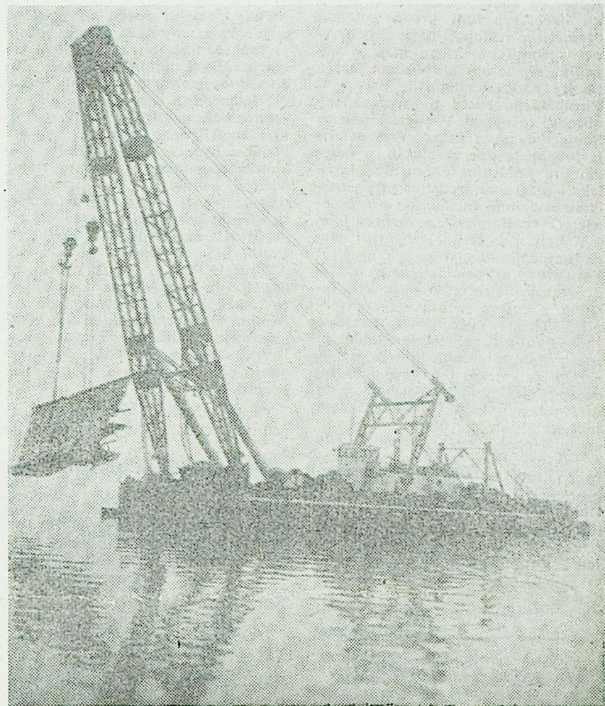
»Veli Jože« pluje s plenom v rokah po morju
