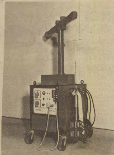
Stroj za sočelno vertikalno varjenje armatur
