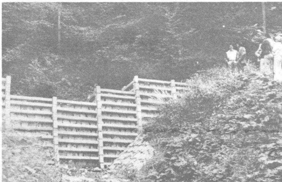
V Žirovnikovem grabnu so delavci Podjetja za urejanje hudoornikov obnovili osem pregrad, ki so narejene iz betonskih kašt. Za tovrstni objekt uporabljajo slovenski izraz »kašta« po celem svetu.
