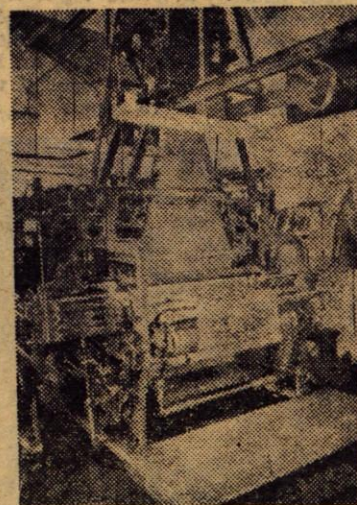
Jacquardski stroj za pletenje svilenih vlaken
