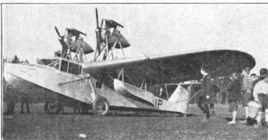
Letalo »Saro Cutty Sark«
