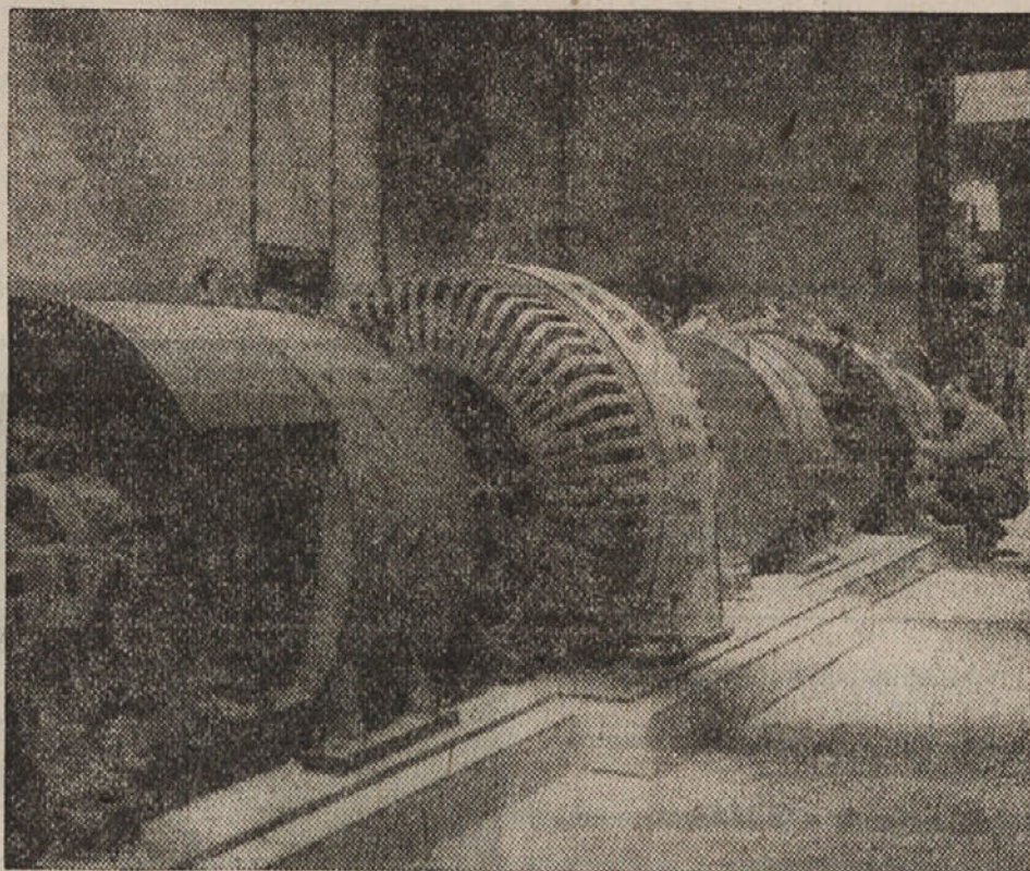
V velikih železarnah v Linzu bodo do jeseni s pomočjo Marshallove pomoči uredili nove valjarne, ki bodo letno proizvajale 300.000 ton valjanega železa. Skupne naprave bodo stale 23 milijonov dolarjev. Na sliki vidimo motorje in generatorje za pogon nove valjarne (USIS).
