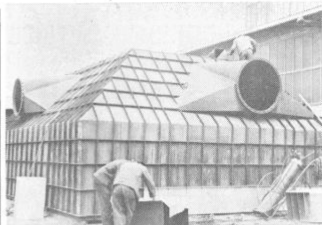
Eden izmed »klobukov«, ki bo lovil pline v novi jeklarni na Ravnah
