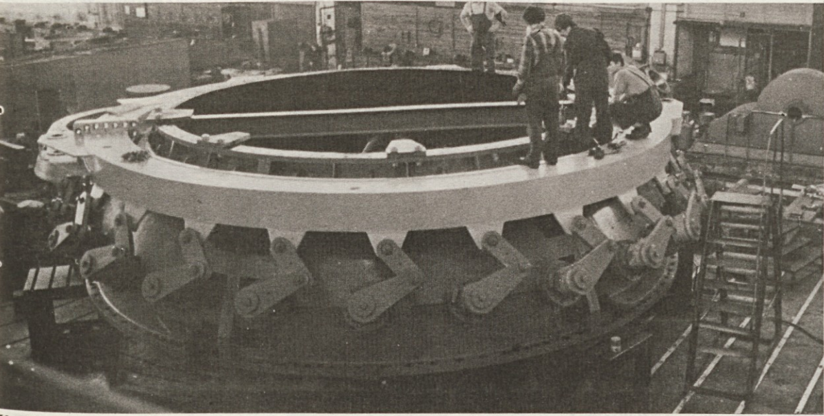
V začetku julija je Litostroj dokončno zapustil prvi konični vodilnik za HE Dubrava. Delavci Montaže na fotografiji izvajajo še zadnje priprave pred transportom na gradbišče. (Foto: T. Š.)
