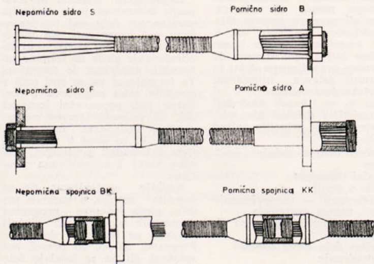
BBRV — kabli z vzporednimi žicami in standardnimi sidri
