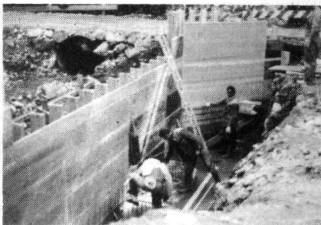
Izgradnja mostu na Srebotnem
