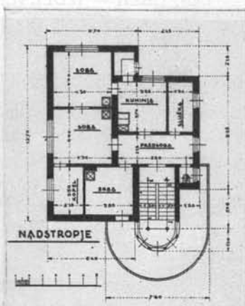
Načrt za dvodružinsko vilo.
