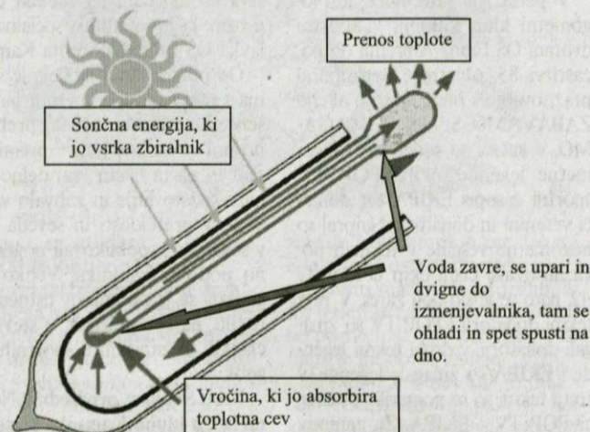
Princip delovanja vroče cevi
