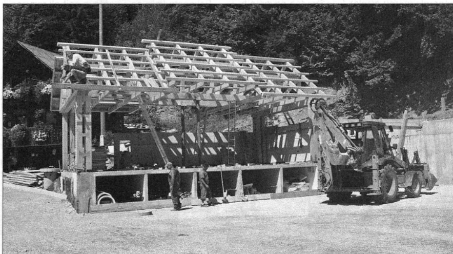
Lesena konstrukcija, kjer bo pokriti oder in servisni prostor za shranjevanje različnih pripomočkov (foto: Marija Lebar)
