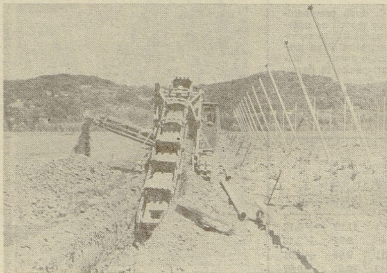
Gradnja namakalnih sitemov je v okviru razvojno-investicijske službe po letu 1965 praktično stekla. Zgrajenih je bilo preko 400 ha naprav
