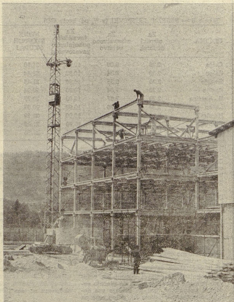
Montažno hmeljsko skladišče je bila prva dokaj drzna rešitev kmetijskega objekta, ki je imela dobre lastnosti, da je bila cena nizka in čas gradnje izredno kratek
