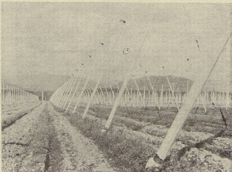
Betonskih hmeljskih žičnic je bilo zgrajenih precej
