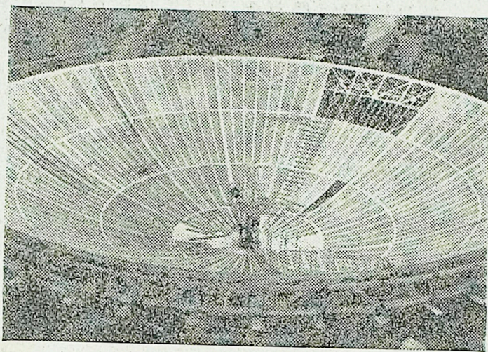
S temle bazenom nameravajo sprejemati iz vse-mirja radijske valove. Kakih 50 kilometrov od Bonna gradijo Nemci naj- bolj sodoben radioteleskop. Reflektor, ki ga vidite na naši sliki meri v premeru nič manj kot 25 metrov.
