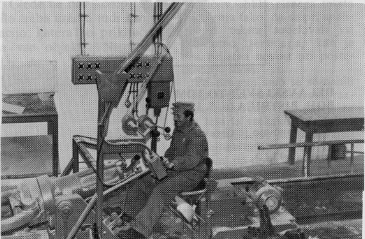
Vpenjalni voziček s komandami za upravljanje polnojarmenika
