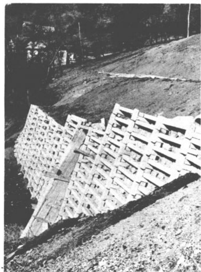
Krajsani Podkraj so se dolgo časa jezili zaradi plazu, ki jim je spodjedal cesto. Sedaj je, kot kaže posnetek, kritična točka odpravljena in cesta je spet varna za promet.
