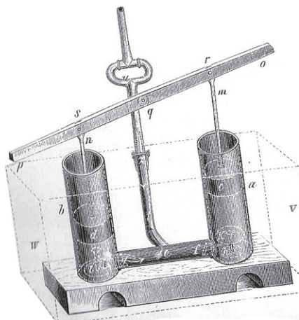
Heronova naprava
