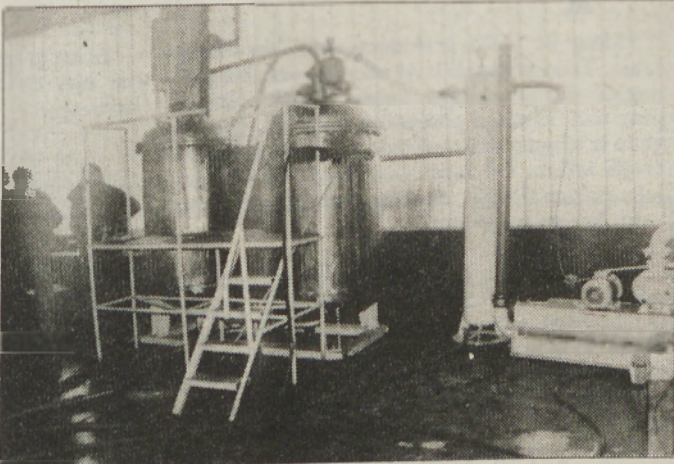
Nemška firma GESUTRA ponuja farmerjem (poleg Nemščaka so zainteresirani tudi druge farne, najbolj pa perutninska farma v Ilirski Bistrici) pri nakupu biološko-mehanske čistilne naprave ugodno posojilo tudi do polovice celotne vrednosti.
