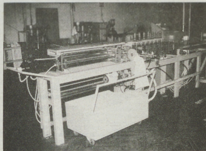
V Elradu so pred kratkim naredili stroj za potrebe paraplegikov v Ljubljani, ki je namensko izdelan in prilagojen potrebam invalidnih ljudi. Upajo, da bo takšnih specialnih naročil v prihodnje več, saj imajo orodje in izkušene delavce, ki jih lahko izpolnijo.
