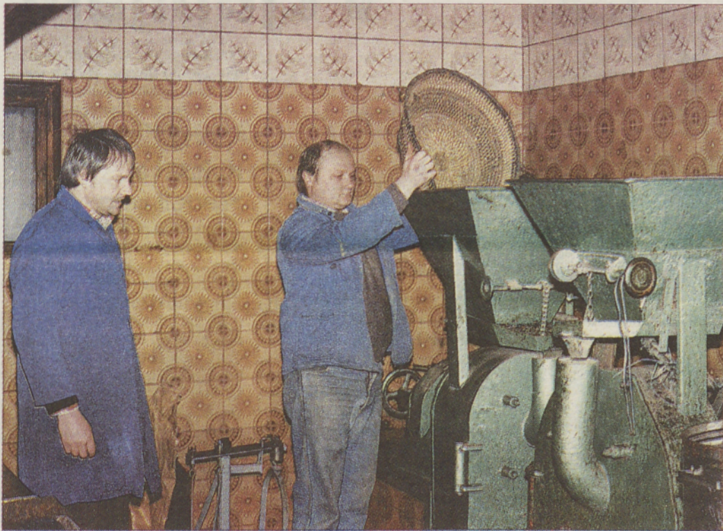
Posušene bučne golice »morajo« najprej v mlin na kamne (ne na valje!). Na levi strani fotografije je Roman Moleh, ki »nadzoruje« vnašanje in delovanje mlina.
