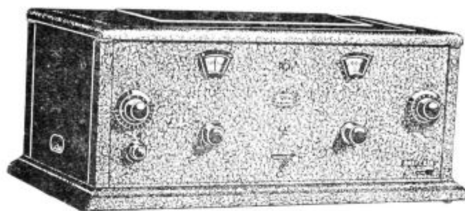
Univerzalni štirielektronski aparat RADIONE za priključek na izmenični tok za KRATKE, NORMALNE in DOLGE VALOVE z elektronkami z zamreženo anodo in vdelano lučno anteno Din 7660—
