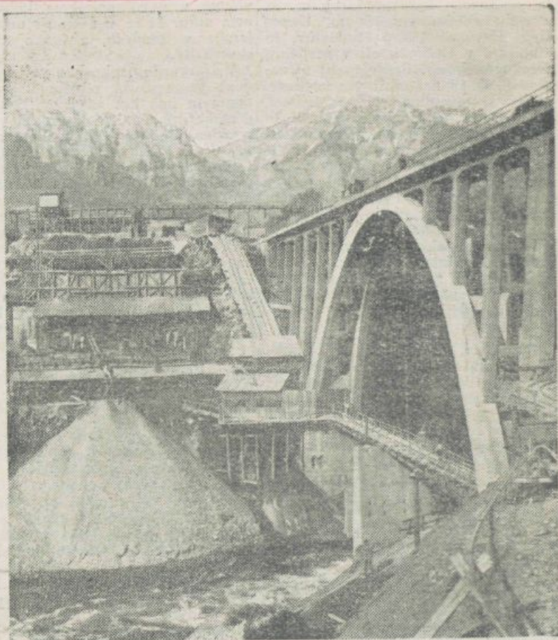
Pri Konjicu bo ozkotirnica speljana na levo obalo Neretve in se bodo Ostrožca na Neretvi toliko dvignila iz doline, da je nastajajoče jezero ne bo poplavelo. Most je moderna gradnja, v enem samem loku je premostil dolino Neretve. Zgradili so ga delavci železniškega gradbenega podjetja s pomočjo frontovskih brigad
