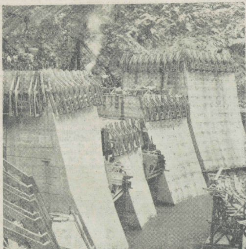
Zb. temiranih je prvih 20 m betonske pregrade, ki bo visoka 75 m ter bo ustvarila jezero dolgo 36 km. V pregrado bo treba vgraditi 170 000 kubinih metrov betona. Centrala bo imela instaliranih 168.000 KW in bo predvidoma letos zabetonirana
