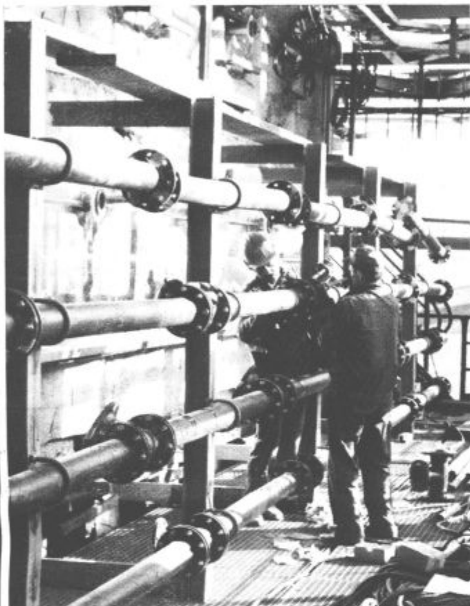
Delo je treba opraviti s popolno natančnostjo. Naprave testirajo s hladnimi zagonskimi preizkusi, šele potem pridejo na vrsto preizkusi z vročim zrakom
