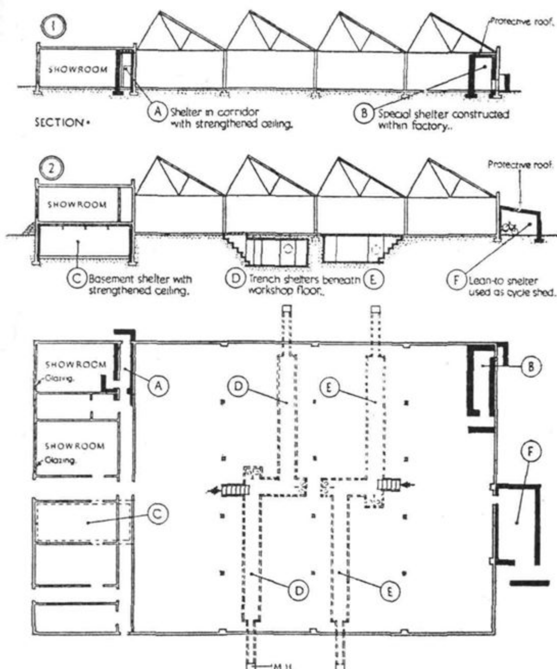
Angleška zavetišča v tovarnah pod in nad zemljo
