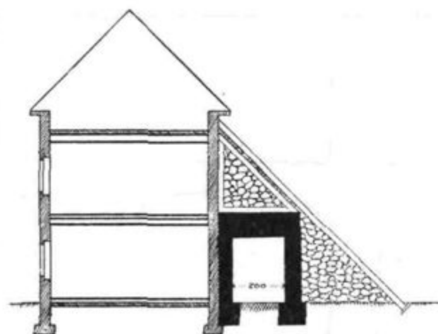
Prerez prislonega zavetišča k hiši, ki ni podkletena
