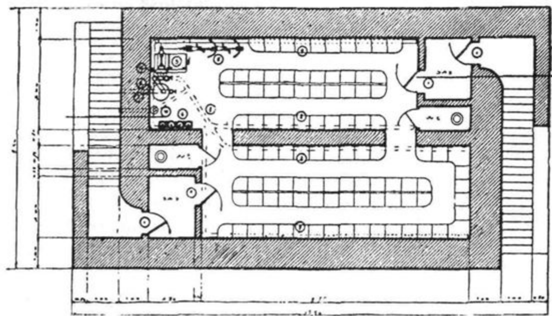
Oklopno zavetišče pod zemljo s prezračevalnimi napravami
