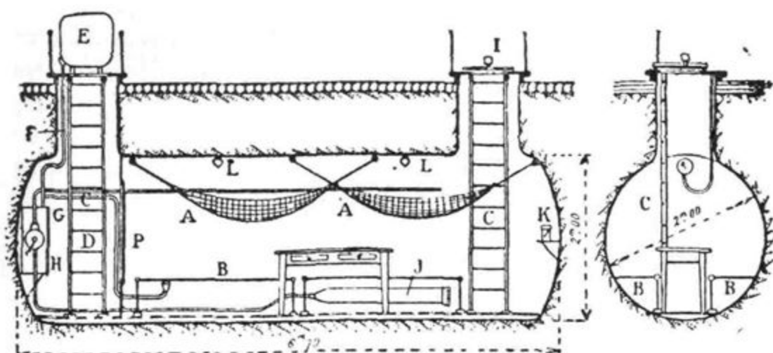
Podolžni in prečni prerez valjastega zavetišča v vlažni zemlji (ing. G. Benoist)
