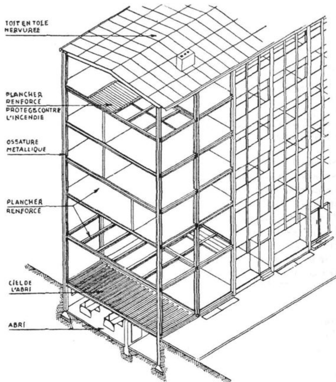
Zasnova zgradbe z jeklenim ogrodjem s posebnim ozirom na zaščito pred zračnimi napadi
