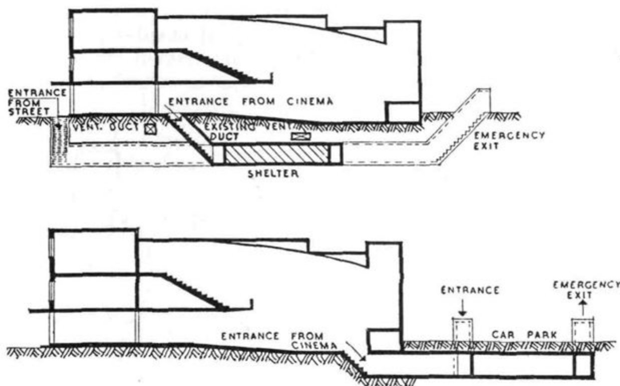
Angleška predloga za zavetišča pri kino dvoranh
