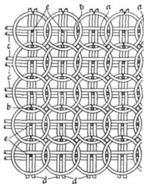
Angleška armatura za stropne oklopne zavetišče
