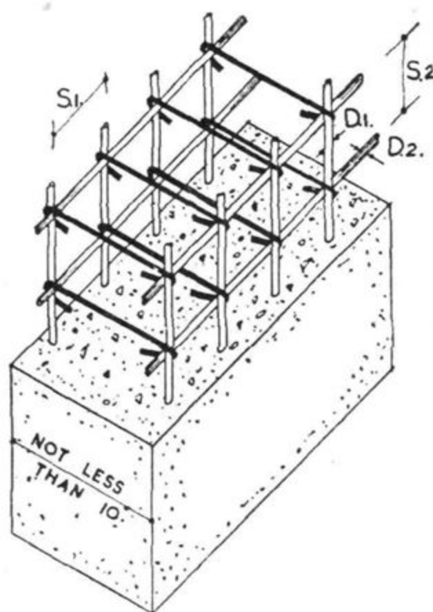
Angleška armatura za stene oklopne zavetišče
