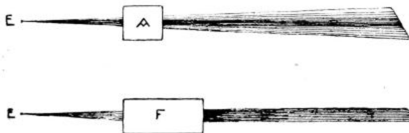
Pregledna slika dejstva običnog akordirajućeg kruga (A) i filtra za propuštanje pruge frekvencije (F) na emisiju moduliranih talasa sa akustičkim tonovima (E).
