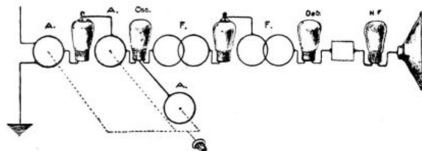
Pregledna šematična slika konstrukcije prijemnika po principu superheterodina. A — akordirajući krugovi, koji se zajednički udešavaju jednim dugmetom za primanje emisije; Osc. — cev detektor-oscilator; F — filter za propuštanje pruge frekvencije konstantne visine; Det. — Drugi detektor; N. F. — niskofrekventna cev.
