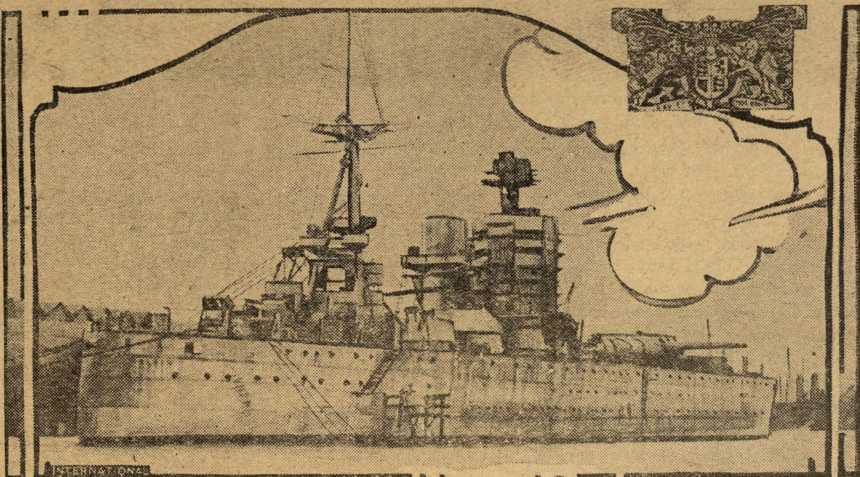
Slika nam predstavlja novo angleško bojno ladjo Nelson, katero z vso naglico gradijo. Ladja bo odplula na poskusno vožnjo v aprilu in bo gotovo kmalu nato pridružena vojnemu brodovju.
