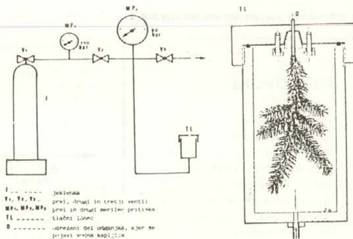
Slika 2: Prikaz »Scholanderjeve bombe« in tlačnega lonca
