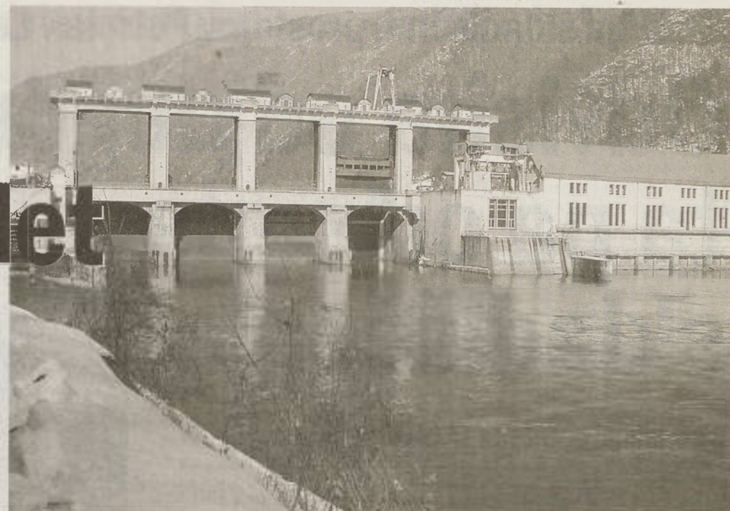
Pogled na HE Fala z desnega brega Drave.
