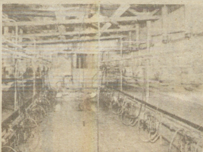
Molzišče za molžo krav tipa „ribja kost“
