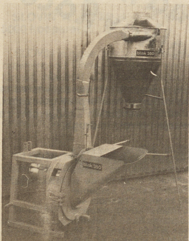
Drobilec za siliranje koruze v zrnju in storžih kapacitete: 2 t/h B 200 E. 8 t/h B 350 S in 15 t/h B 500 S.
