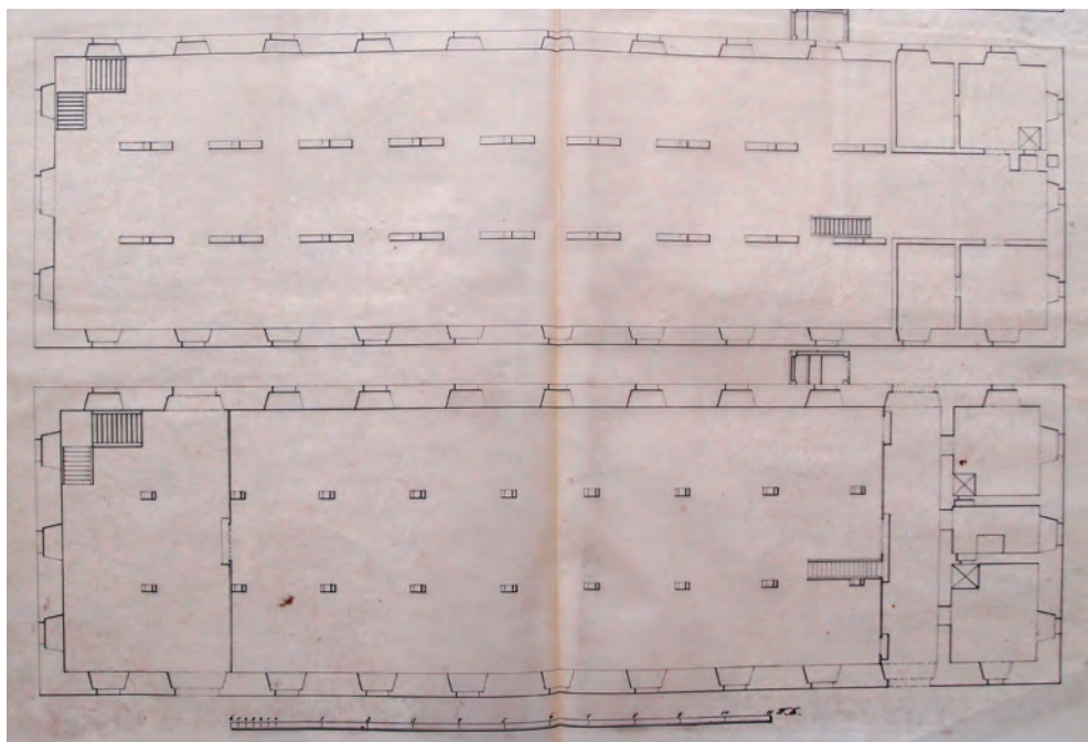
123. Načrt notranjosti idrijskega skladišča (Si AS 50, Gradbena direkcija, š. 279).
