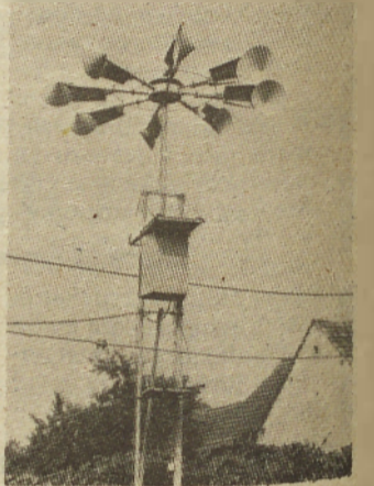
Vetrnica na dvorišču Hasa Gaberca, ki jo poganja veter, polni akumulator. In ko zmanjka toka, je potreben samo pritisk na gumb in iz dveh žarnometov posije dovolj močna svetloba, da lahko tudi ponoči bere.
