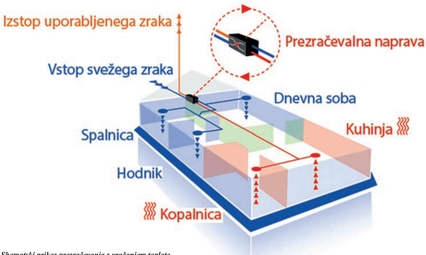
Shematski prikaz prezračevanja z vračanjem toplote
