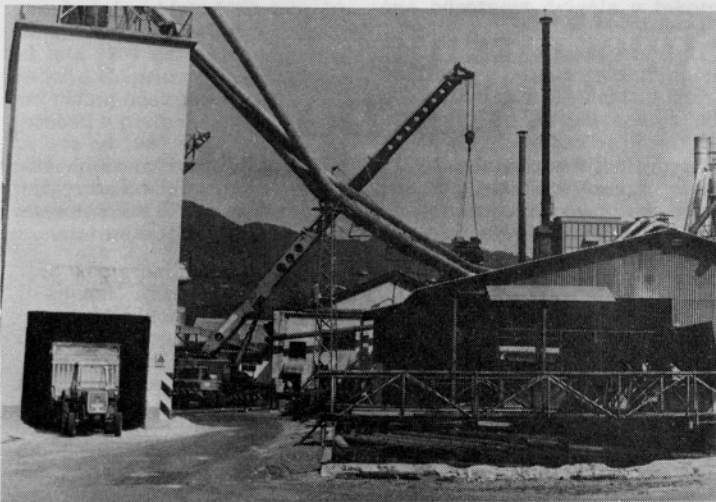
Spuščanje polnojarmenika skozi streho žage na temelje
