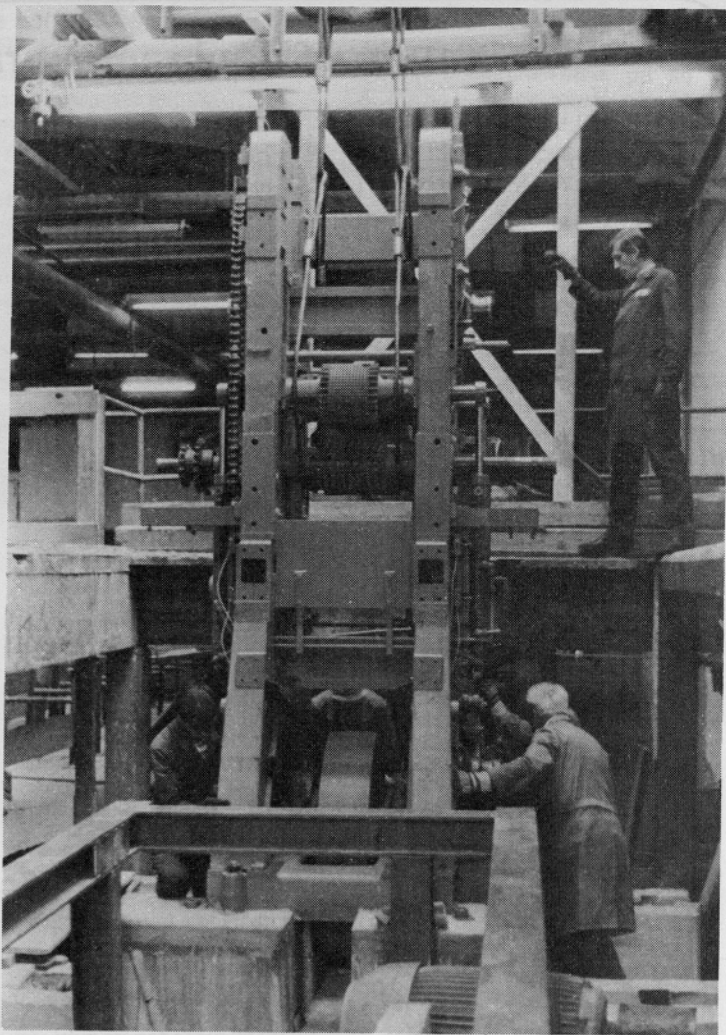
Montaža polnojarmenika
