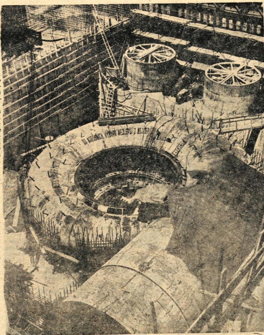
Gradnja ene največjih hidrocentral na Češkoslovaškem
