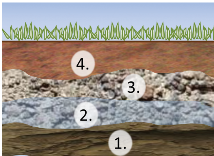
Prečni prerez zemeljske plasti: 1 = plast gline, 2 = plast podtalnice in proda, 3 = plast proda, 4 = plast prsti.
