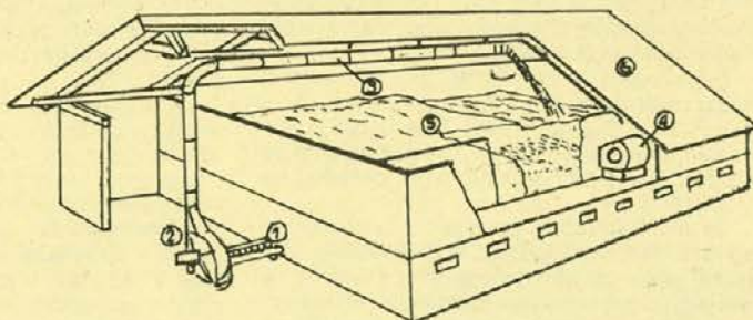
SONČNI SENIK Z LINIJO ZA TRANSPORT ZA SUŠENJE SENA
