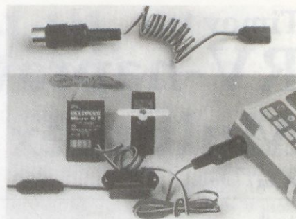
Slika 6. Diagnostični kabel ali po domače zveza brez radijskih valov.
