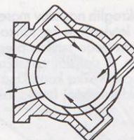
Risba 4. Tangencialno izpiranje
