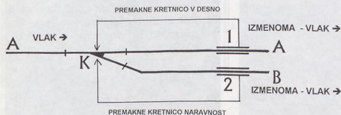
Ko vlak prevozi kontaktni tir 1 ali 2, premakne kretnico v odklon ali naravnost.
