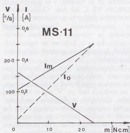
Risba 5. Lastnosti servomehanizma MS 11 – največji navor znaša 25 Ncm
