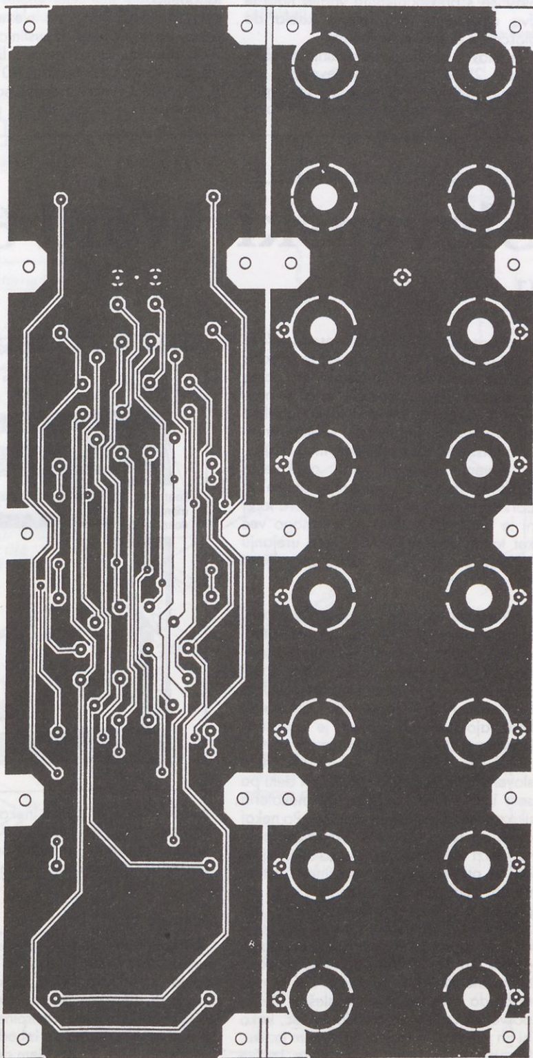
Risba 2. Ploščica tiskanega vezja
