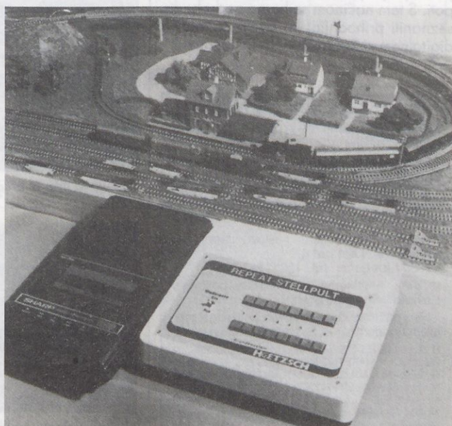
Elektronska upravljalna omarica s kasetnikom omogoča avtomatsko nastavitve vnaprej izbrane vozne poti.
