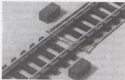
Reed kontakt je tako majhen, da ga lahko vgradimo v tir namesto praga. Ob strani sta dva magneti. Magnet pritrdimo na spodnjo stran vozila.
