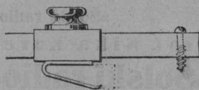
37. slika. Gibljiv kontakt na vodilni palici.
