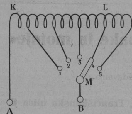
38. slika. Večdelna tuljava, pri kateri se samoindukcijska da z ročico M in kontaktnimi gumbi 1 do 5 izpreminjati. V naznačeni legi ročice je tuljavin del K—L zvezan s privijali A in B.
