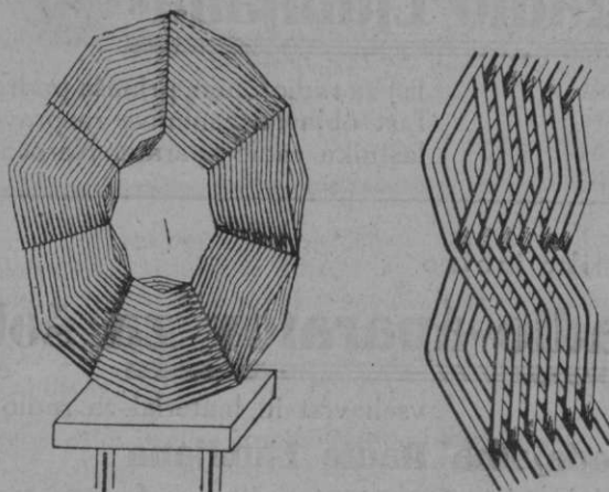
42. slika. Tuljava v obliki dna košare; poleg del ovojev povečan.
