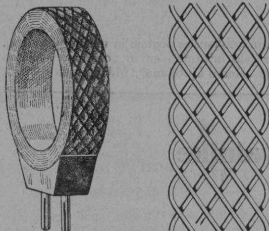
41. slika. Satovna tuljava, poleg nje del ovojev močno povečan.
