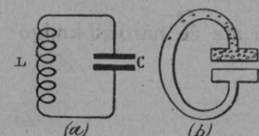
35. slika. Nihajni krog (a), ki obstoja iz tuljave L in kondenzatorja C, primerjamo lahko z dvema sobama (b), ki sta zvezani po dolgem hodniku.
