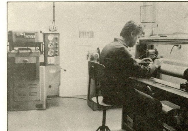
Priprava — montaža valjev za tisk na anilinskih strojih
