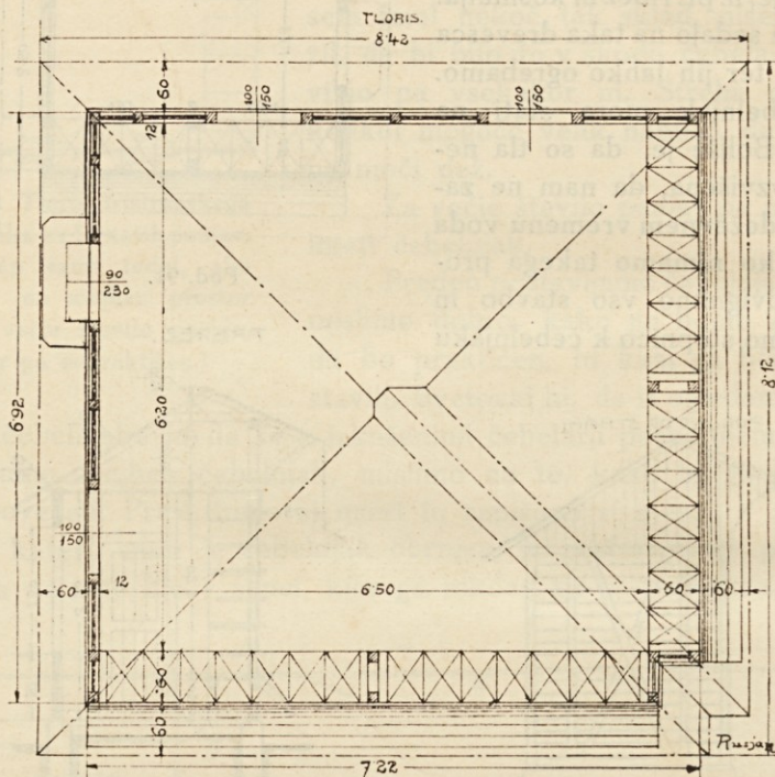
Pod. 94. Dvostranski čebelnjak za 84 naših panjev. (Tloris.) (Praktična oblika za majhen prostor in v olepševalne svrhe.)
