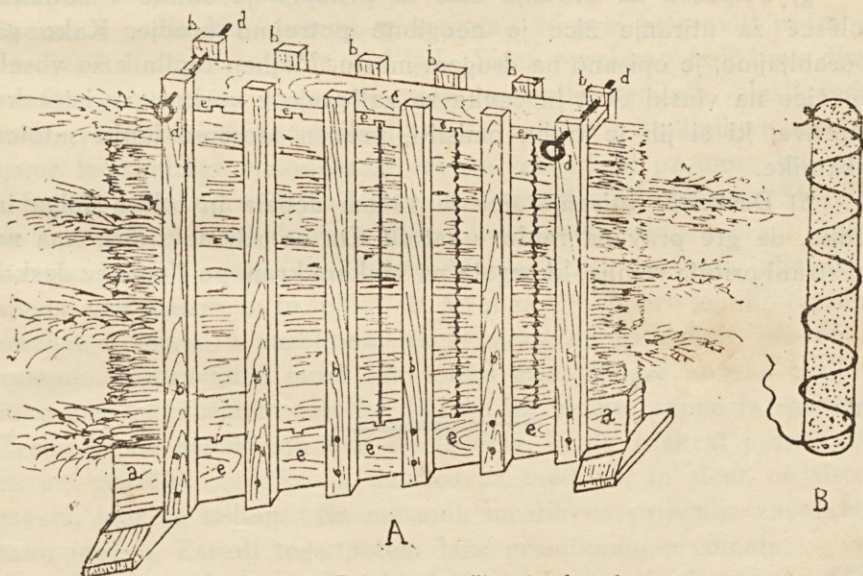
Pod. 53. Priprava za šivanje slamnic.
