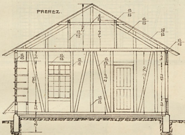
Pod. 95. Dvostranski čebelnjak za 84 naših panjev. (Prerez.)
