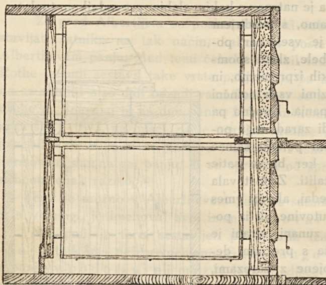
Pod. 3. Podolžni pokončni prerez.
