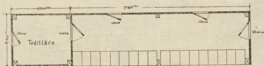
Pod. 90. Tloris enostranskega čebelnjaka s trčališčcem za 54 naših panjev. Po tem načrtu je zgrajen moj zunanji čebelnjak v Ribnici pri Ilir. Bistrici. (Najbolj praktična oblika čebelnjaka.)
