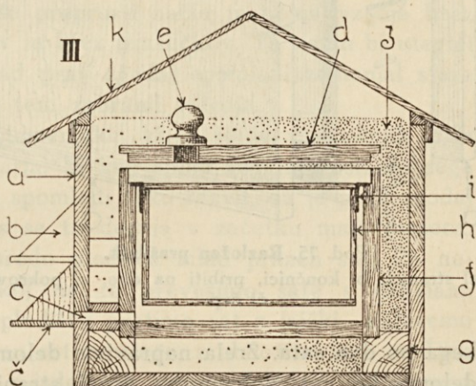
Pod. 74. Pokončni prerez skozi prašilnik.
