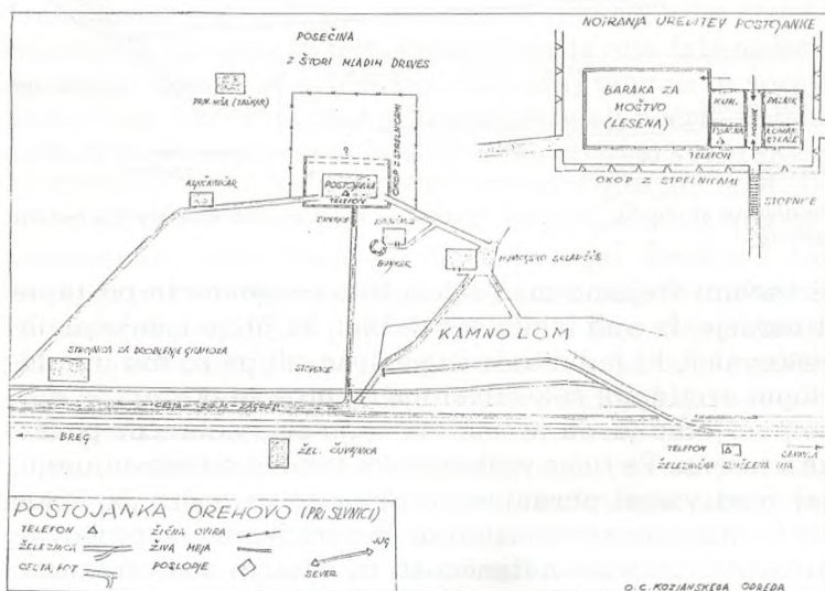
Skica postojanke OrehoVo — izdelek obveščevalnega centra odreda.
