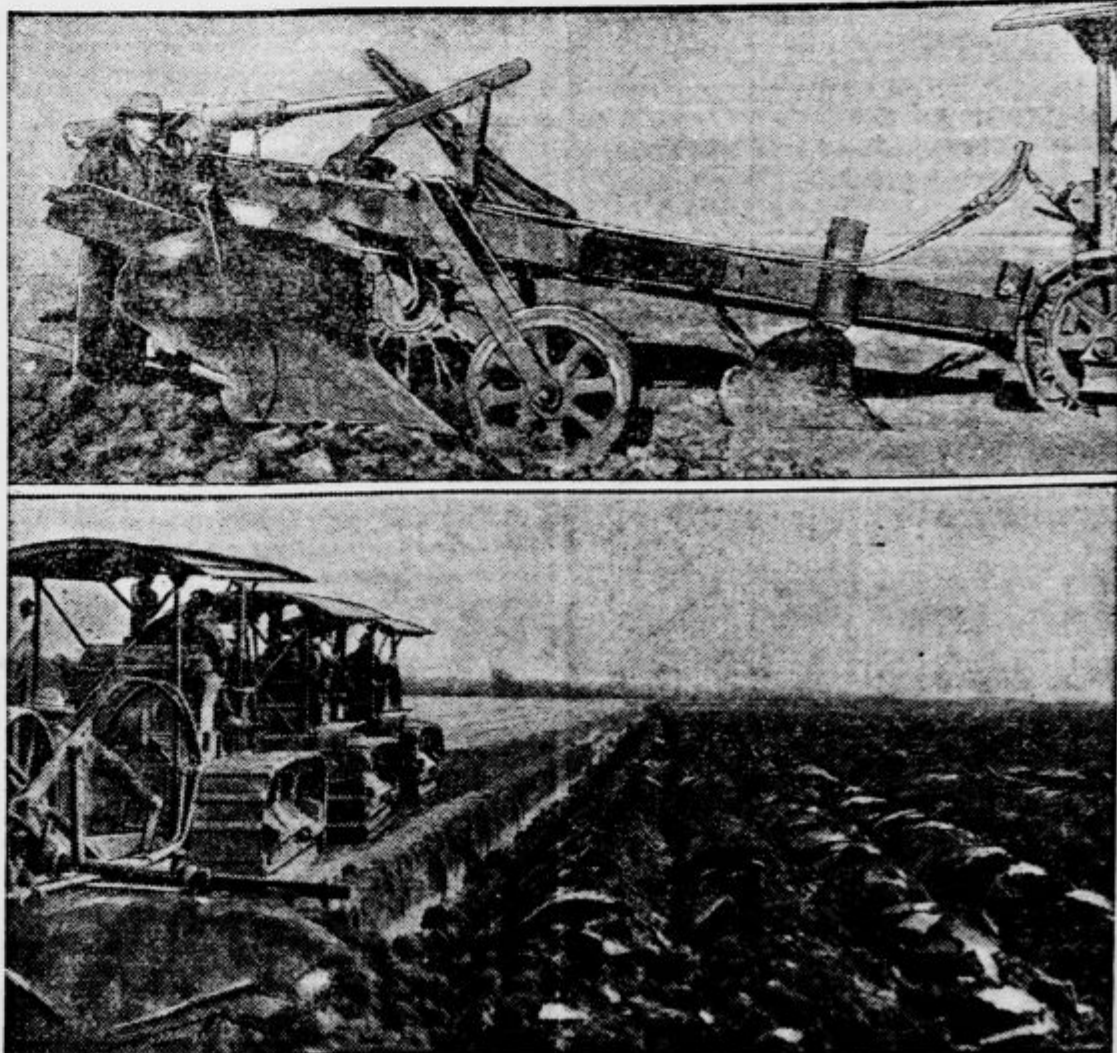
Zgoraj: Ogromen plug, čigar velikost se vidi zlasti iz primerjave človeka na levi. Spodaj: Trije traktorji, ki so potrebni za vlačenje pluga, ki reže 1 m globoke in 90 cm široke brazde.
