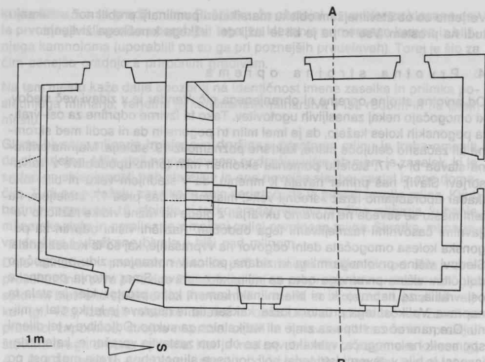
Sl. I. Tloris pritličja sedanje stavbe
